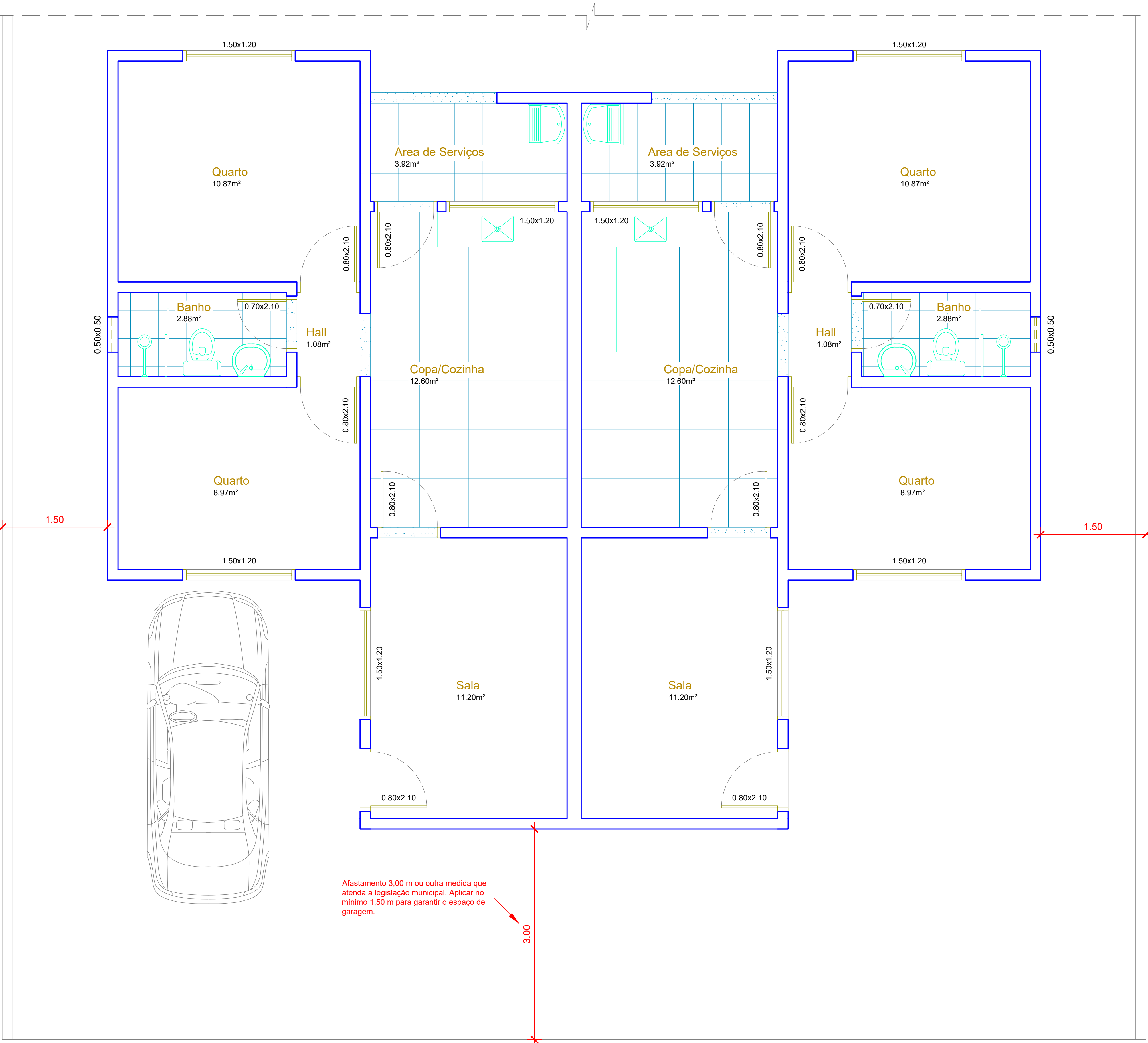
PLANTA BAIXA - IMPLANTAÇÃO GEMINADA
